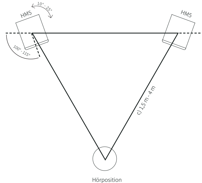
Abbildung 10. HM5 - Aufstellung - Stereodreieck.
