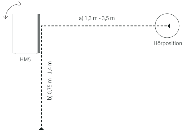
Abbildung 11. HM5 - Aufstellhöhe.
