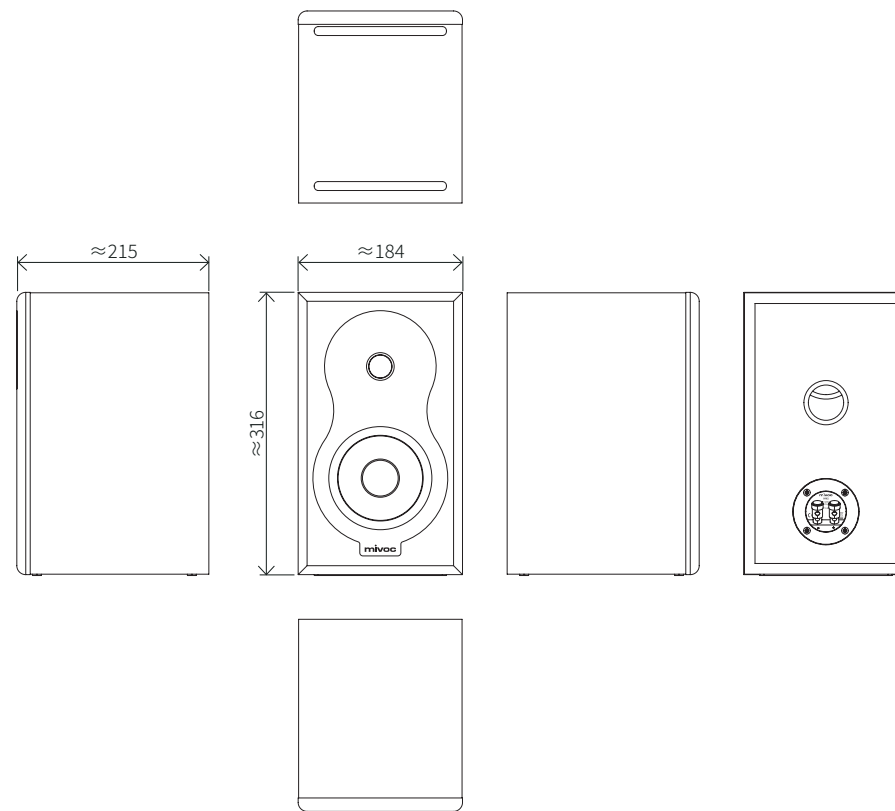
Abbildung 13. HM5 - technische Zeichnungen.
