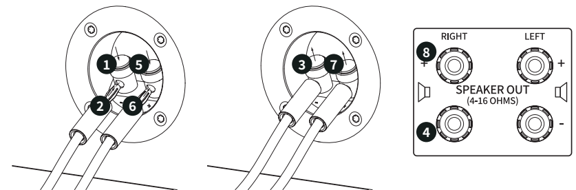
Abbildung 8. HM5 - Anschluss Lautsprecherkabel (mit Stecker).
