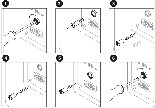
图 9.AM 80MKII - 更换保险丝。
