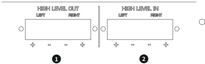
图 3.AM 80MKII - 高电平输入/输出。
