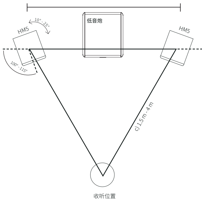
图 11. 使用 AM 80MKII 自制的低音炮 - 安放。
