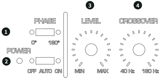
图 5. AM 80MKII - 系统设置。
