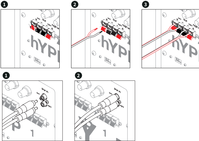
图 10.AM 80MKII 和 hYPE 10G2 扬声器和音频电缆接口。
